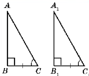
Рис. 149. Прямоугольные треугольники ABC и A_1B_1C_1 равны по катету и прилежащему острому углу
