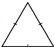
Рис. 82. Равносторонний треугольник
