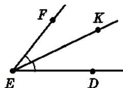
Рис. 22. Луч EK — биссектриса угла DEF
