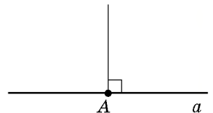
Рис. 69. От любой полупрямой прямой a можно отложить прямой угол
