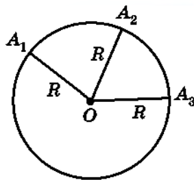
Рис. 162. Расположение точек плоскости, удаленных от точки O на расстояние R
