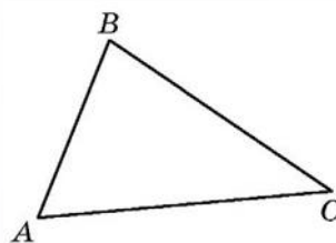
Рис. 54. Треугольник ABC
