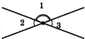
Рис. 40. Углы, смежные с одним и тем же углом, равны
