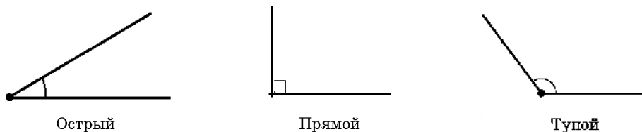
Рис. 25. Виды неразвернутых углов
