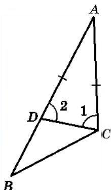
Рис. 156. К доказательству соотношений между сторонами и углами треугольника
