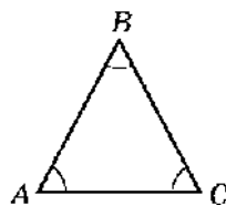
Рис. 86. К признаку равностороннего треугольника
