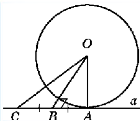
Рис. 168. К доказательству свойства касательной
