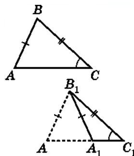
Рис. 61. Две стороны и угол двух треугольников соответственно равны, но сами треугольники не равны
