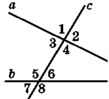
Рис. 118. Прямая c пересекает прямые a и b
