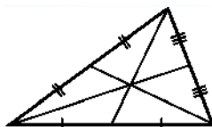
Рис. 96. Три медианы треугольника пересекаются в одной точке
