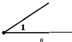
Рис. 17. Обозначение угла
