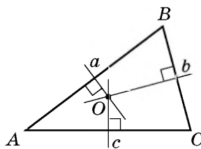
Рис. 184. Точка O — точка пересечения серединных перпендикуляров к сторонам треугольника ABC
