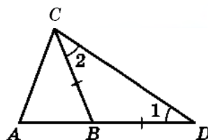
Рис. 157. К доказательству неравенства треугольника
