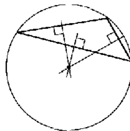
Вне треугольника
