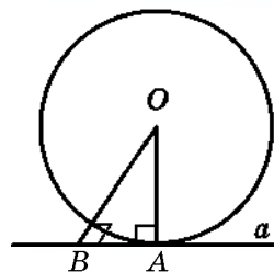
Рис. 169. К доказательству признака касательной
