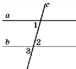
Рис. 121. \angle 1 = \angle 3 , тогда a \parallel b
