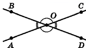
Рис. 44. При пересечении двух прямых образуются две пары вертикальных углов
