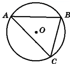
Рис. 183. Окружность, описанная около треугольника ABC
