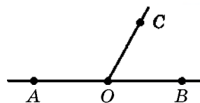
Рис. 35. Углы AOC и COB смежные
