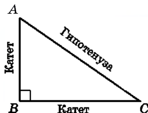
Рис. 147. Прямоугольный треугольник
