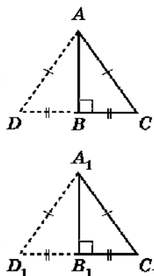
Рис. 152. Прямоугольные треугольники ABC и A_1B_1C_1 равны по гипотенузе и катету
